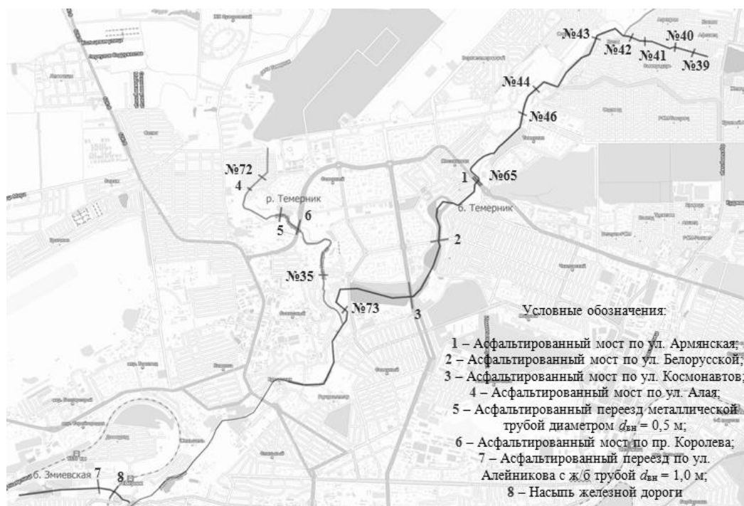
Рисунок 2 – Плановая схема расположения мостов и переездов
