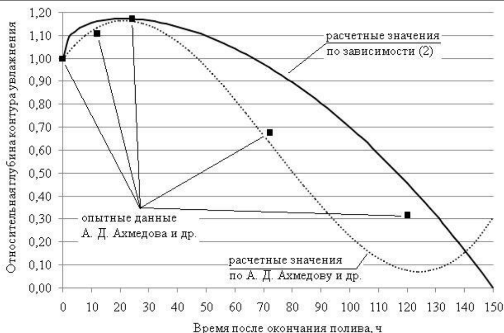
Рисунок 3 – Значения относительной глубины контура каплевого увлажнения, полученные по зависимости (2), по первичным данным и по уравнению А. Д. Ахмедова для W_{г/ч} = 77,5 \% МСП
