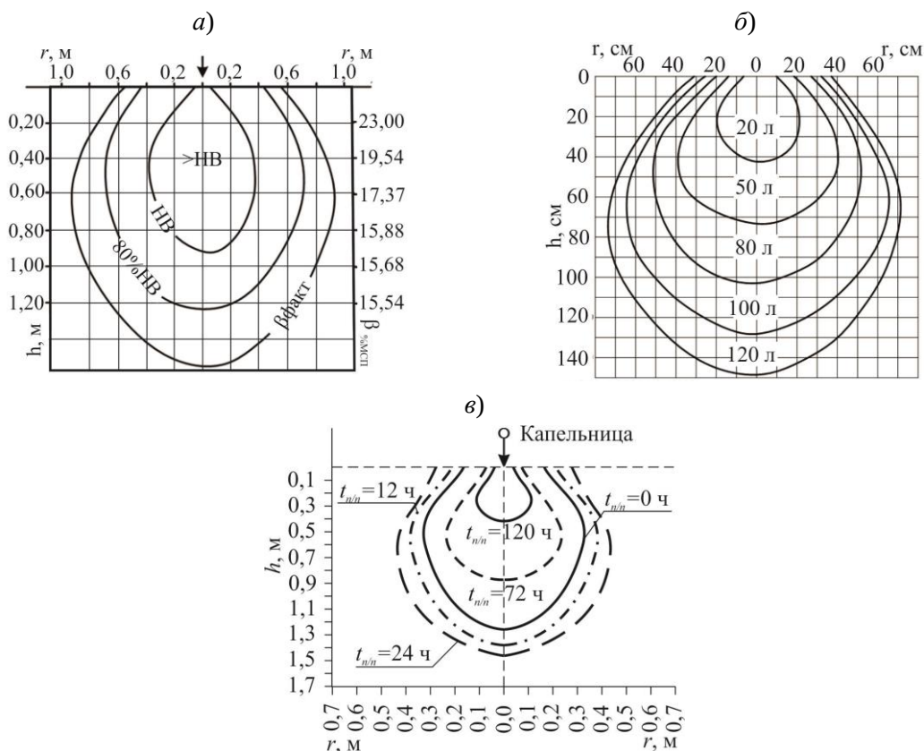
а) по данным О. Е. Ясонида [3]; б) по данным А. Д. Ахмедова и др. [4]; в) по данным В. С. Бочарникова [5]
