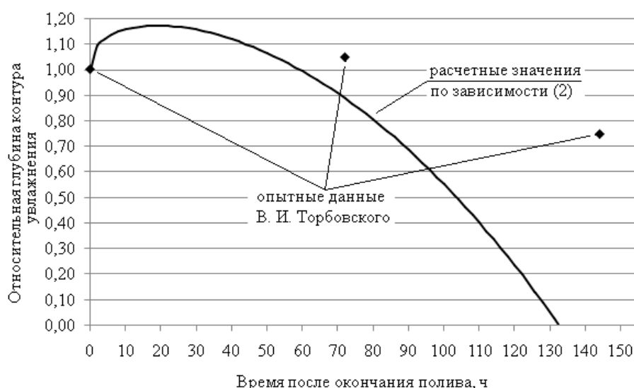
Рисунок 4 – Значения относительной глубины контура каплевого увлажнения, полученные по зависимости (2) и по первичным данным В. И. Торбовского для W_{г/ч} = 64,8 \% МСП
