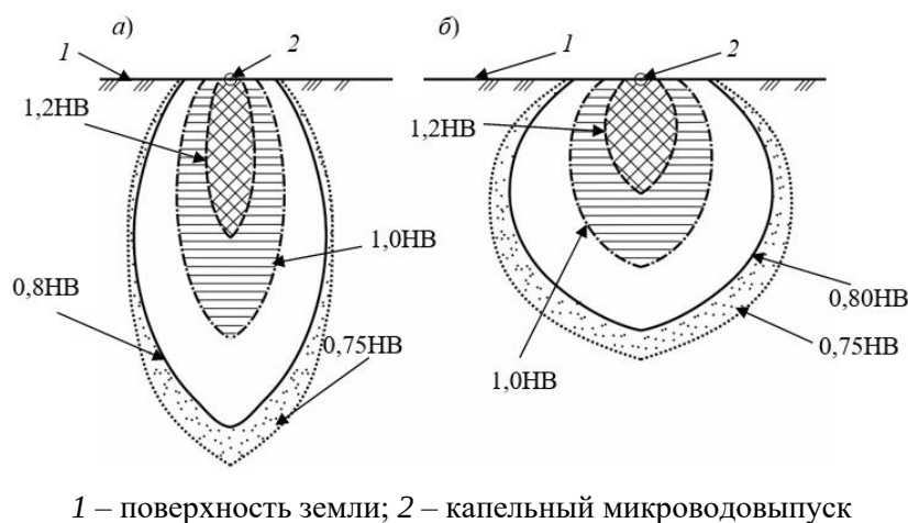
Рисунок 1 – Схемы контуров увлажнения, формируемых в почвогрунтовом пространстве при капельном поливе в песчаных (а) и в глинистых (б) почвах
