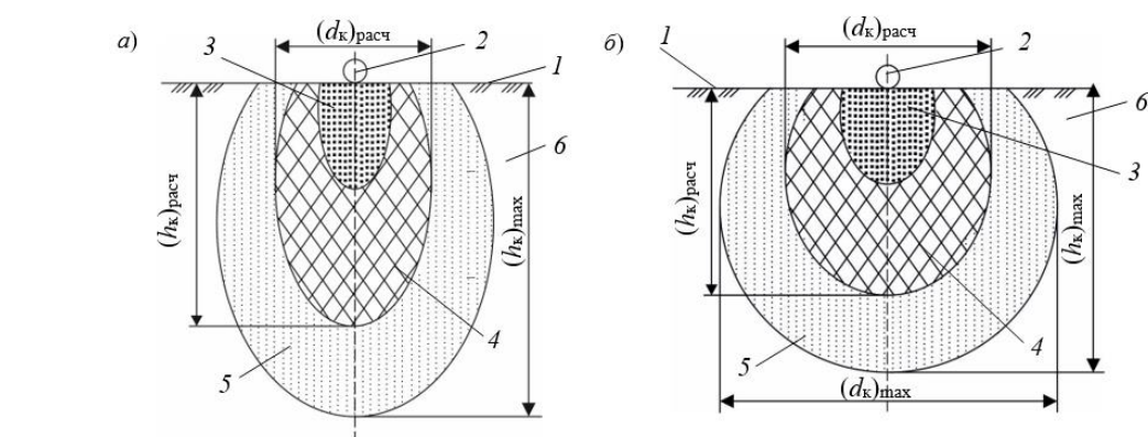
а) на песчаных почвах; б) на глинистых почвах; (d_k)_{расч} – расчетный диаметр контура; (h_k)_{расч} – расчетная глубина контура; (d_k)_{max} – максимальный диаметр контура; (h_k)_{max} – максимальная глубина контура; 1 – поверхность земли; 2 – капельница наземного расположения; 3 – переувлажненная зона; 4 – зона (область) расчетной влажности; 5 – зона недостаточного увлажнения; 6 – зона естественного увлажнения
