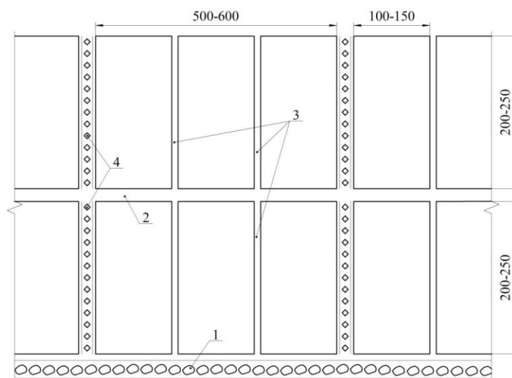
1 – садозащитная лесная полоса; 2 – межкуартальная (внутрисадовая) дорога; 3 – внутриквартальная междоузельная дорога; 4 – межкуартальная защитная лесополоса (размеры в метрах)
