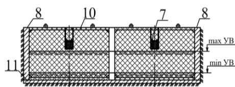
Разрез Д – Д
