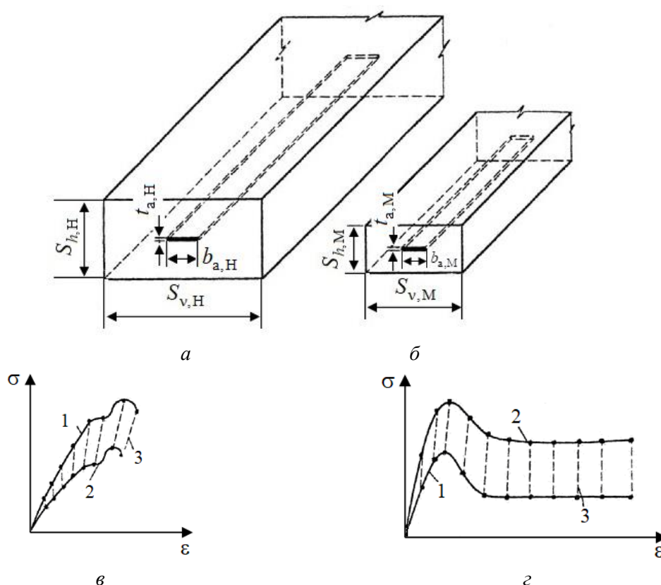
a и б – армированный грунт соответственно натуре и модели; в – подобие индикаторных диаграмм для металлической арматуры; г – подобие индикаторных диаграмм для пластмасс и синтетических материалов; 1, 2 – индикаторные диаграммы соответственно натуре и модели; 3 – линии сходственных напряжений
